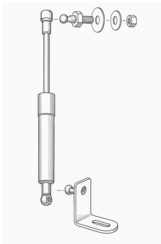
Haubenlift MB 907
